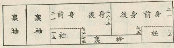
並幅1米80糎(四尺八寸)にて 裾廻しの裁ち方並に裁ち切り寸法
