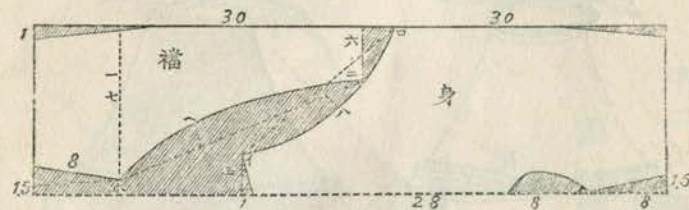
並幅65糎(一尺七寸)にて 寝冷え知らず(二-三歳用)の裁ち方並に裁ち切り寸法
