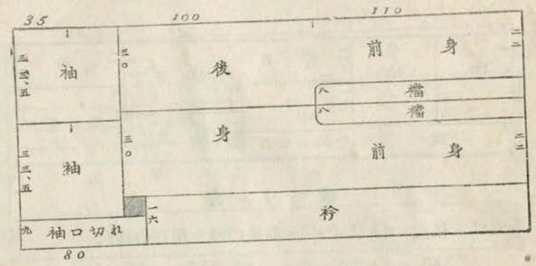
76糎(二尺)幅にて 元祿袖中裁羽織の裁ち方並に裁ち切り寸法
