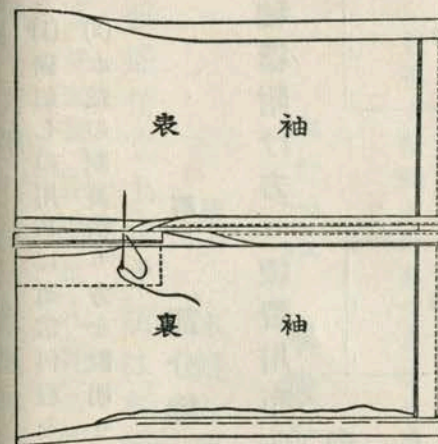
袖口・振りの綿含め方
