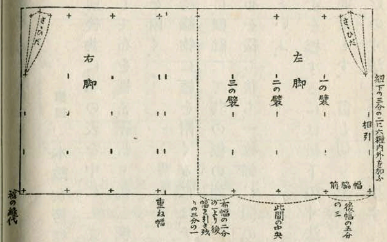
女袴前布の標付け方
