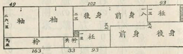
第一圖 三つ身單衣の裁ち方並に裁ち切り寸法
