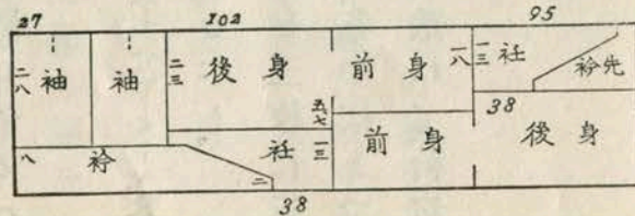
第二圖 筒袖三つ身單衣の裁ち方並に裁ち切り寸法
