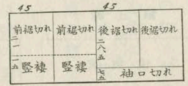
並幅1米80糎(四尺八寸)にて 裾廻しの裁ち方並に裁ち切り寸法
