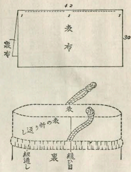
羽衣手提の縫ひ方
