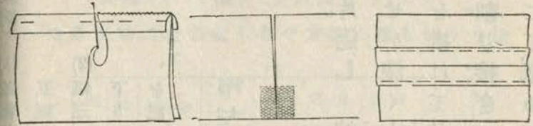
掛け接ぎ 突合せ接ぎ 割り接ぎ
